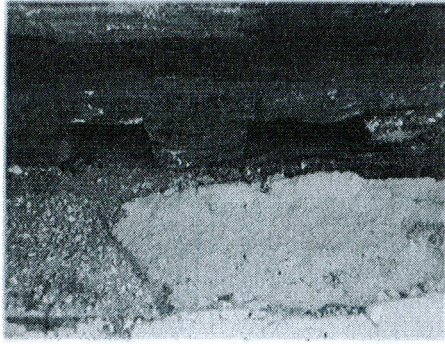
لایه‌های رسوبی در نزدیکی سد
